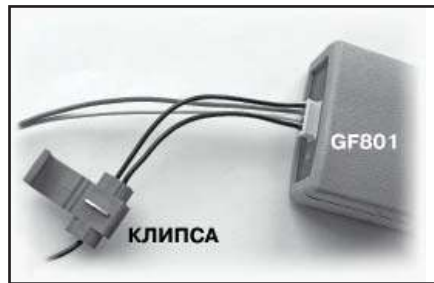
Рис.4. Подключение парктроника.
